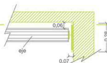
vista corte A-A / ESC. 1:20
