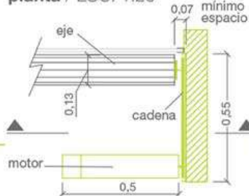
planta / ESC. 1:20
